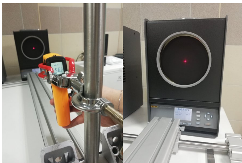
Stanowisko do wzorcowania pirometrów
